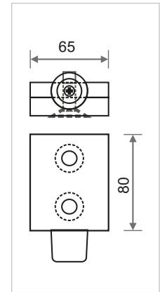
Endanschläge Rollco® LWS 125
